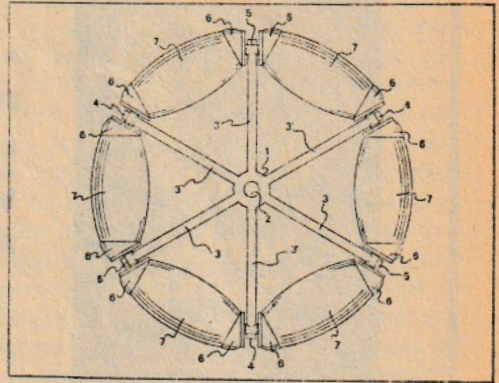
Her yöne hareket edebilen tekerlek. NASA tarafından onaylanmış olan patenti Müh. Josef F. Blumruch'e aittir.
